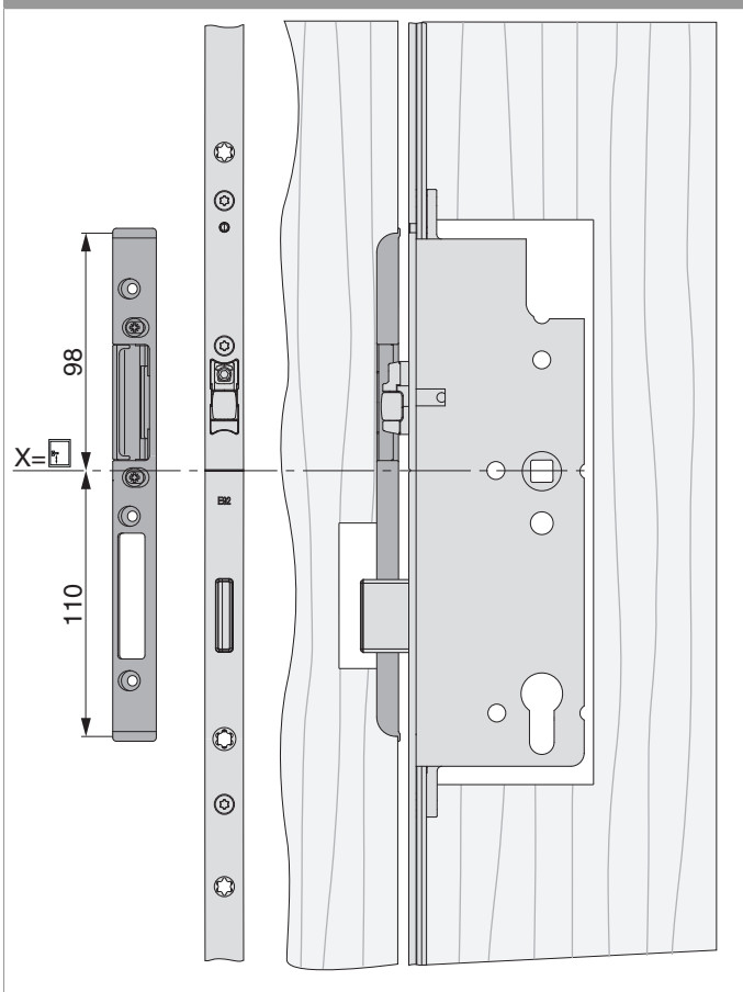
Schließteile Rollfalle
